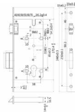
AML-8550/MR Mortise Roller
