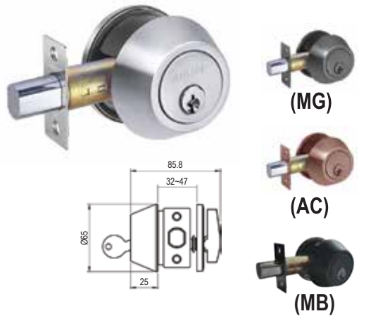
ADL-101 Thumbturn & Key Deadbolt
