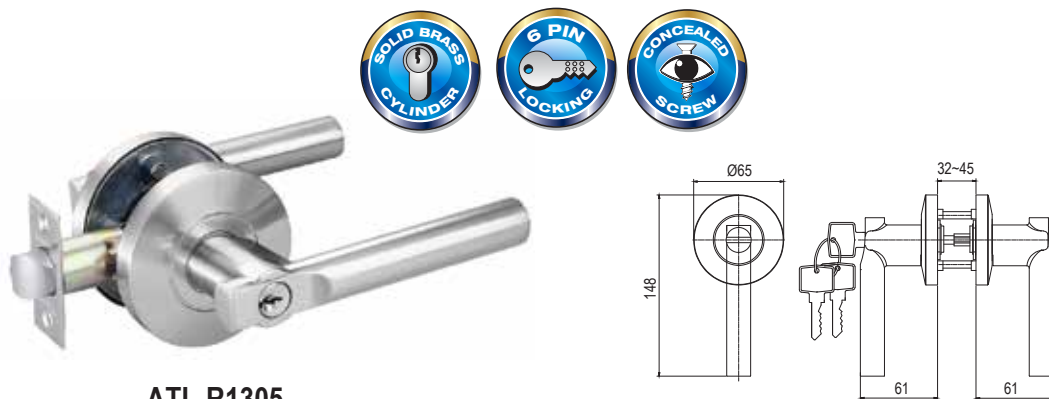
ATL-R1305 Tubular Lever
