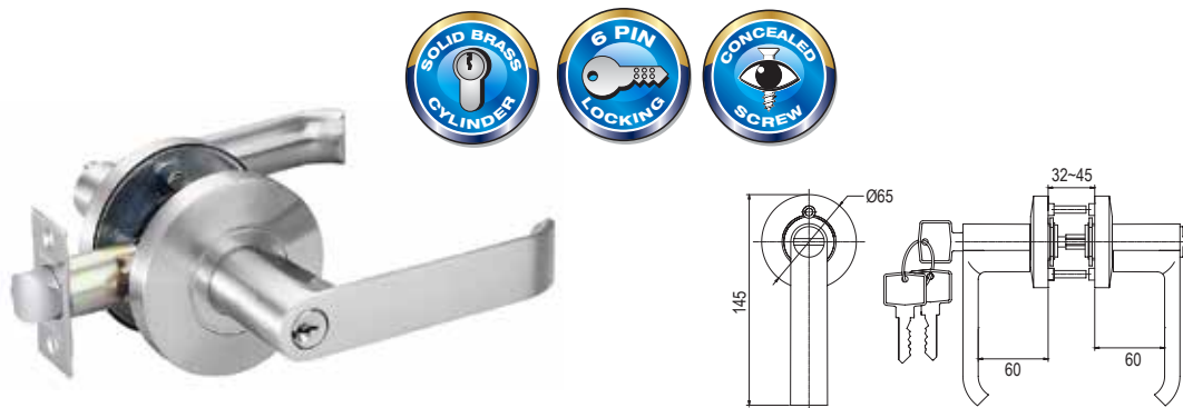
ATL-R1303 Tubular Lever
