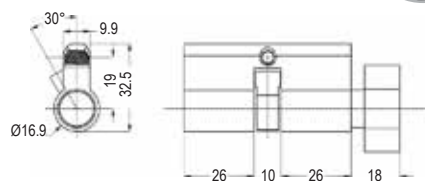
APC-AS/MB Key & Thumbturn
